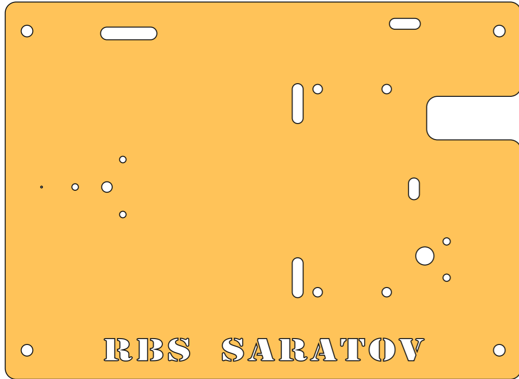
04-003 Верхнее основание робота 1 шт.
