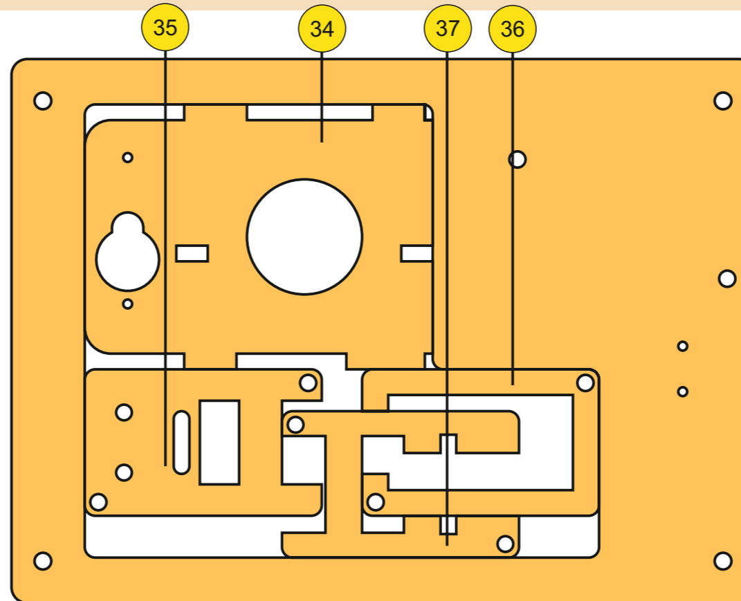
04-0042 Нижнее основание робота 1 шт.
